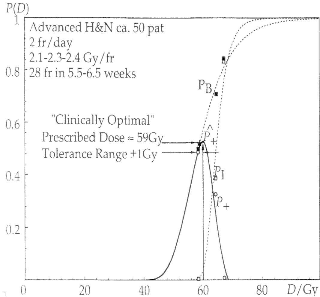
Fig. 1 - Relações dose-efeito estabelecidas clinicamente para tumores avançados da cabeça e pescoço (" Specification of dose delivery in Radiation Therapy ", Recommendations by the Nordic Association of Clinical Physics, NACP (1994))
