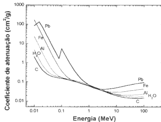
Fig. 3 Coeficiente massa de atenuação
