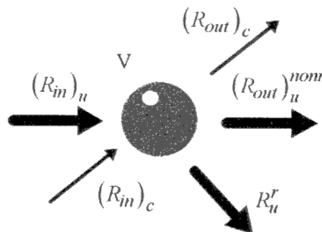
figura 3 - Esquema correspondente ao termo de balanço de energia \varepsilon , a partir do qual se define dose absorvida.
