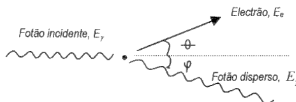
Fig. 1 – Efeito Compton
